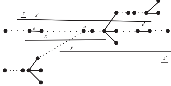
Figure 16. T UV-model; lab(e) \not\subseteq lab(e') , lab(e') \not\subseteq lab(e) and lab(e) \cap lab(e') \neq \emptyset .
