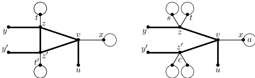
Figure 9. Cases F1 and F2 for Lemma 3.4.
